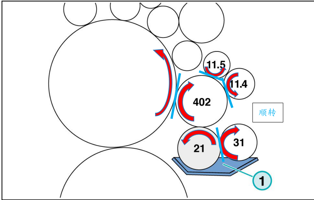
罗兰 R700 水路结构
