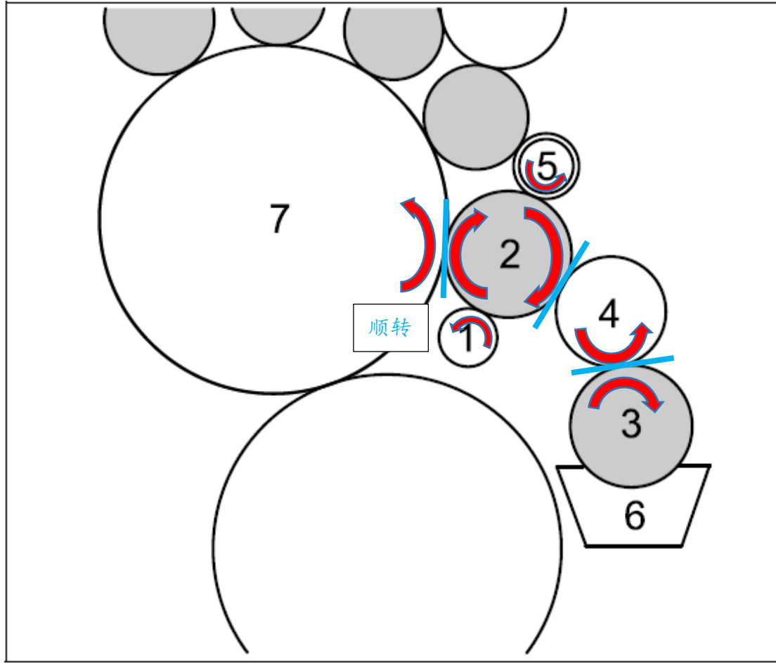
高宝 RA106 水路结构
