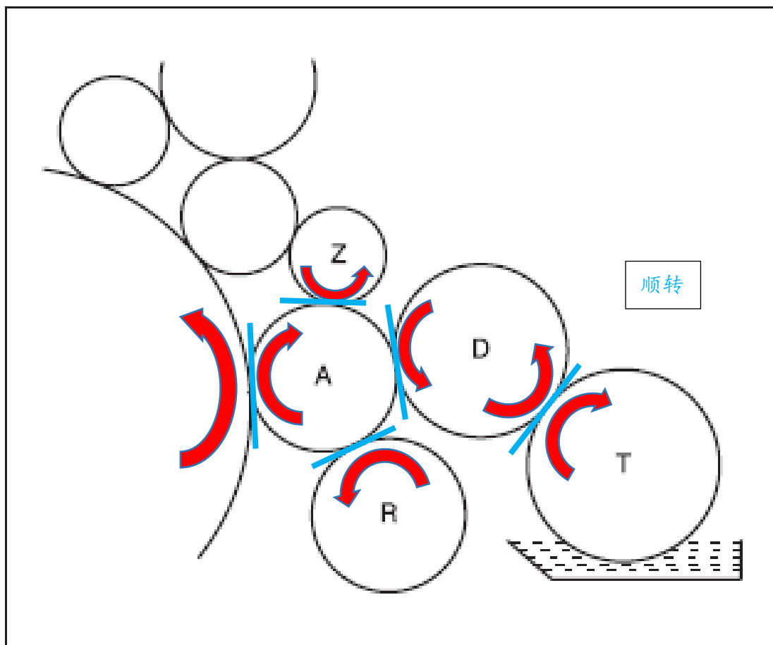
海德堡 CD102 水路结构
