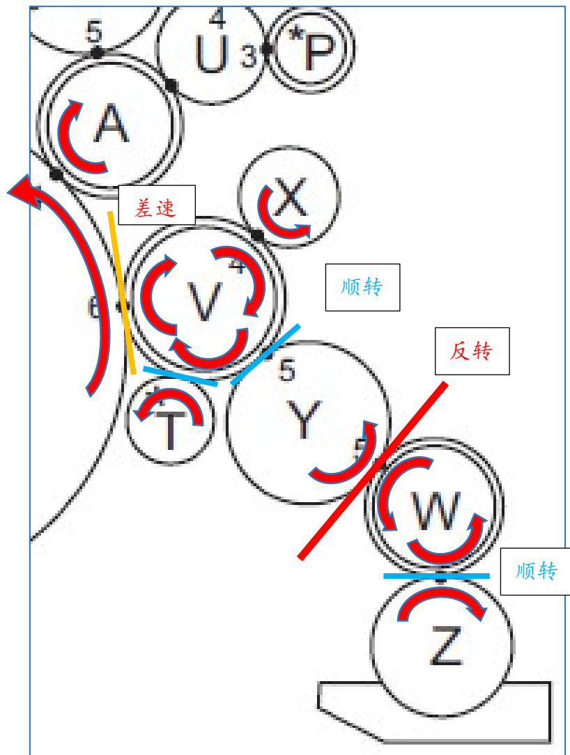
小森 GL-40 水路结构
