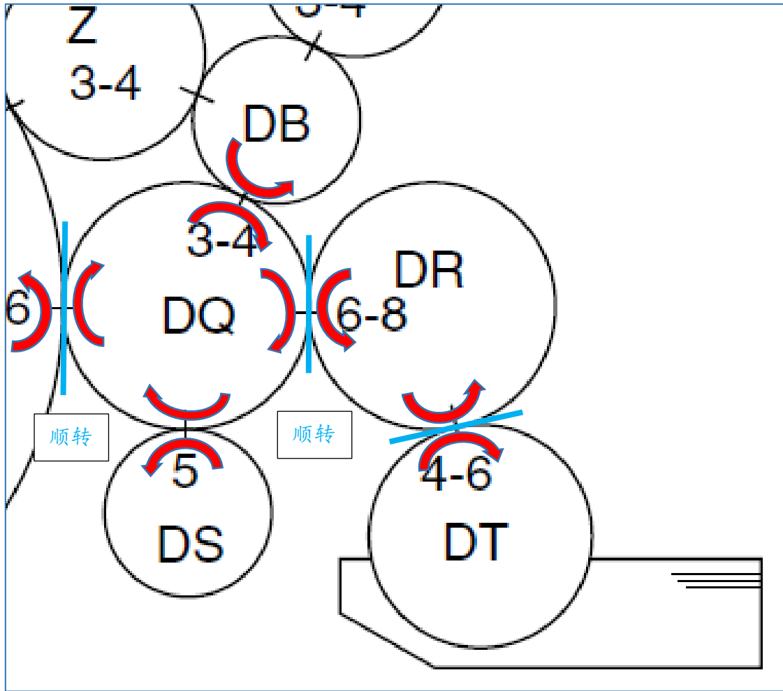
新菱 RMGT 10 水路结构
